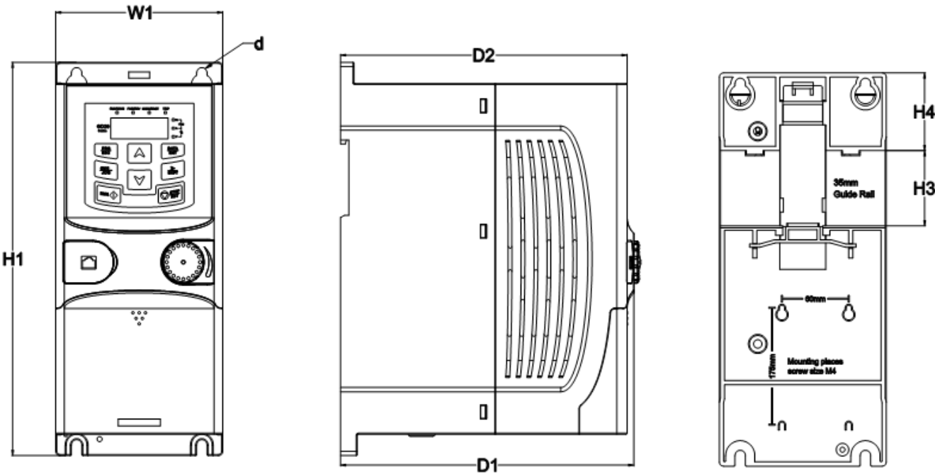
Montage sur rail des variateurs de 1PH 200 V/3PH 380 V (≤2.2 kW) et 3PH 200 V (≤0.75 kW) Dimension (unité : mm)
